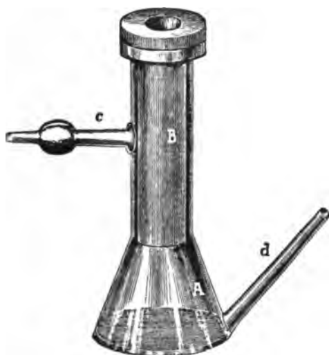
FIG. 11.—Reichel filter.
